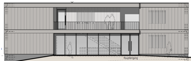
Abbildung 2: Nord-Ansicht mit Haupteingang
