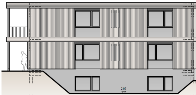
Abbildung 1: Ost-Ansicht mit Werkstatt & Atelier
